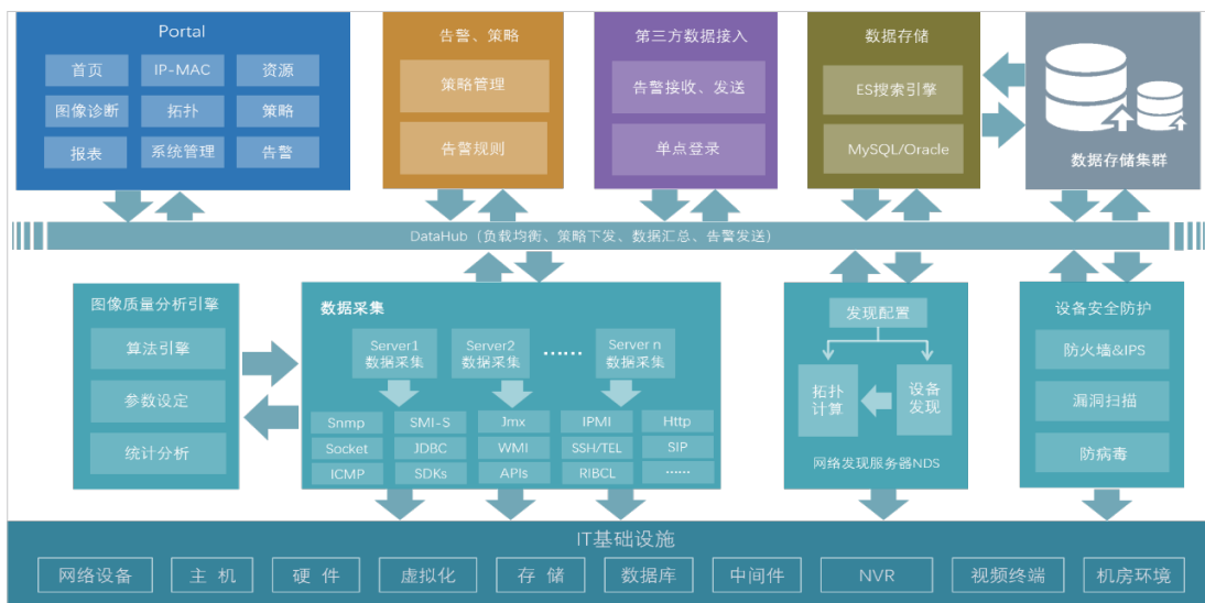
图 1 智慧运维安全管理平台架构
