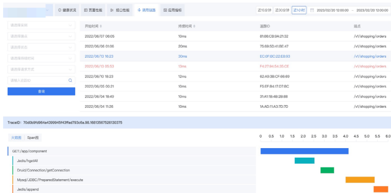
图8 系统调用链路
