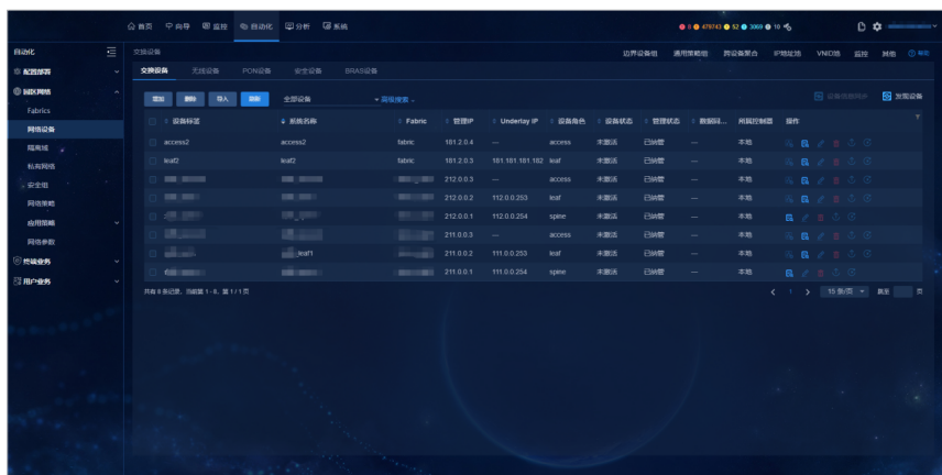
图 4 配置模板
