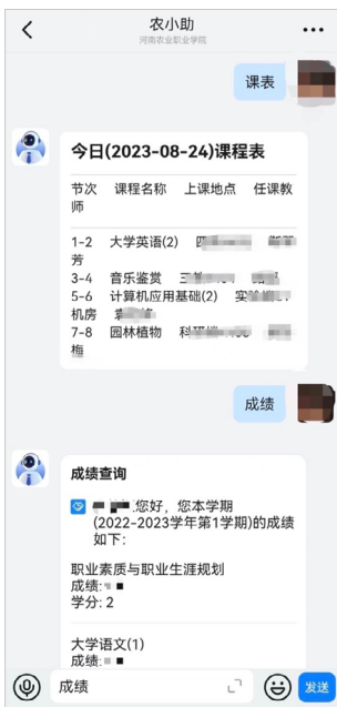
图 5 数据服务
