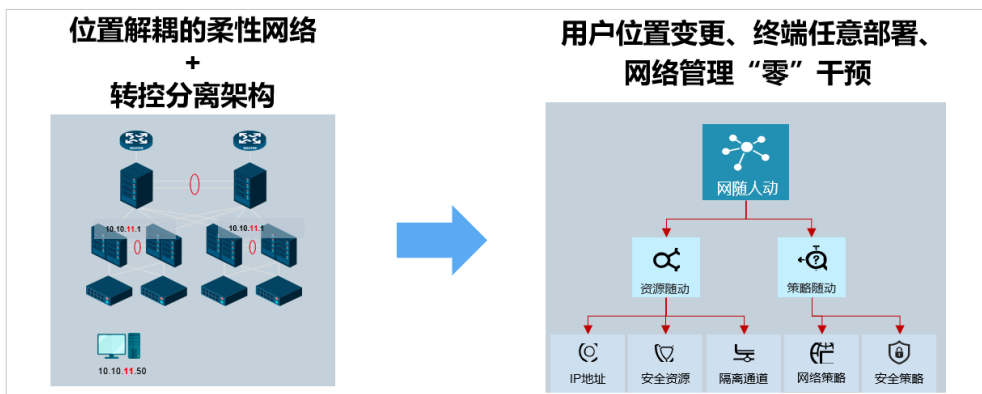
图 5 网随人动
