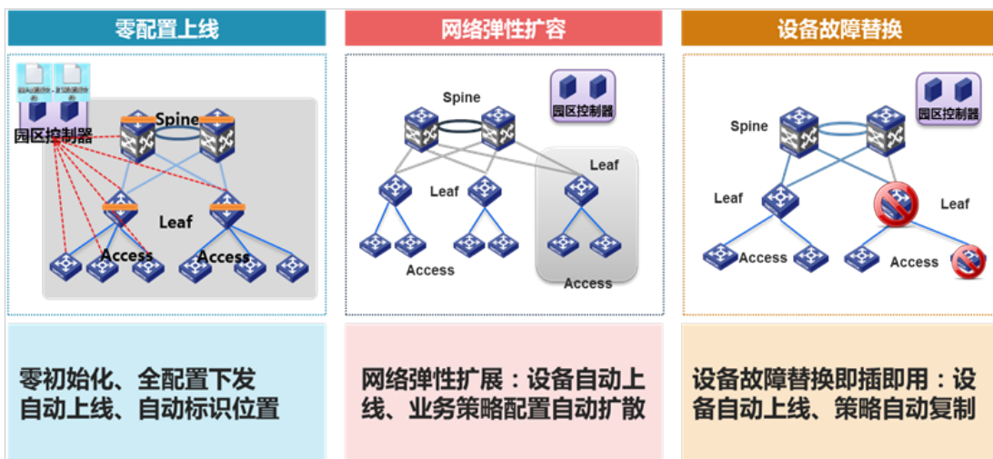
图 1 零配置上线
