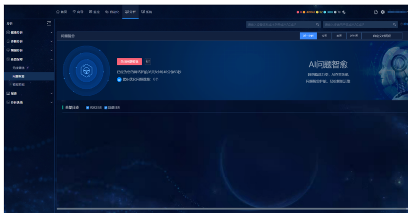
图 9 故障自愈
