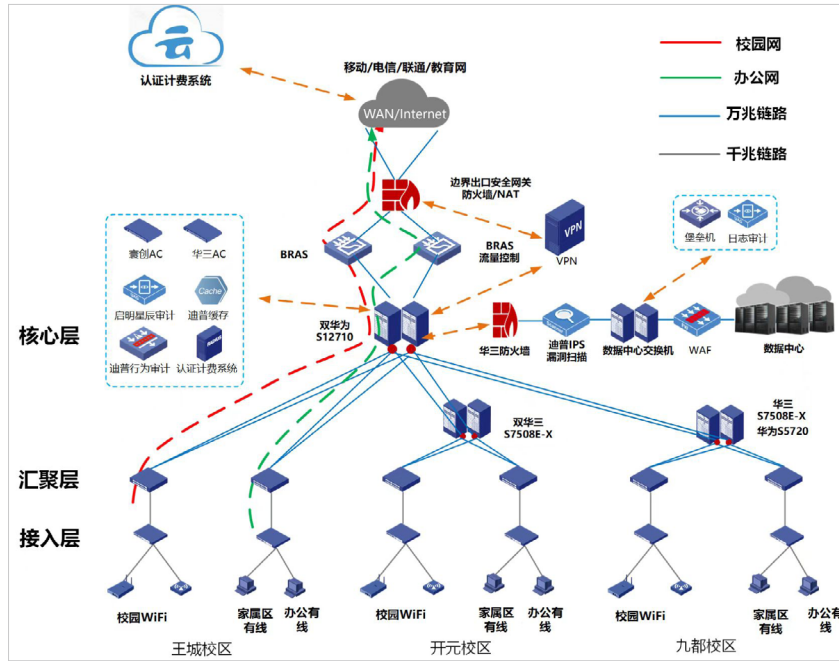
图 1 洛阳理工学院校园网拓扑结构
