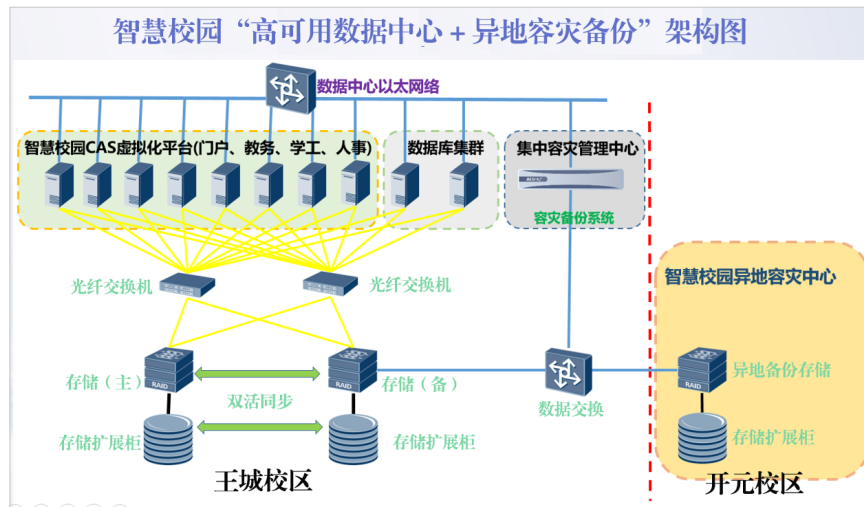
图 2 洛阳理工学院高可用数据中心 + 异地容灾系统
