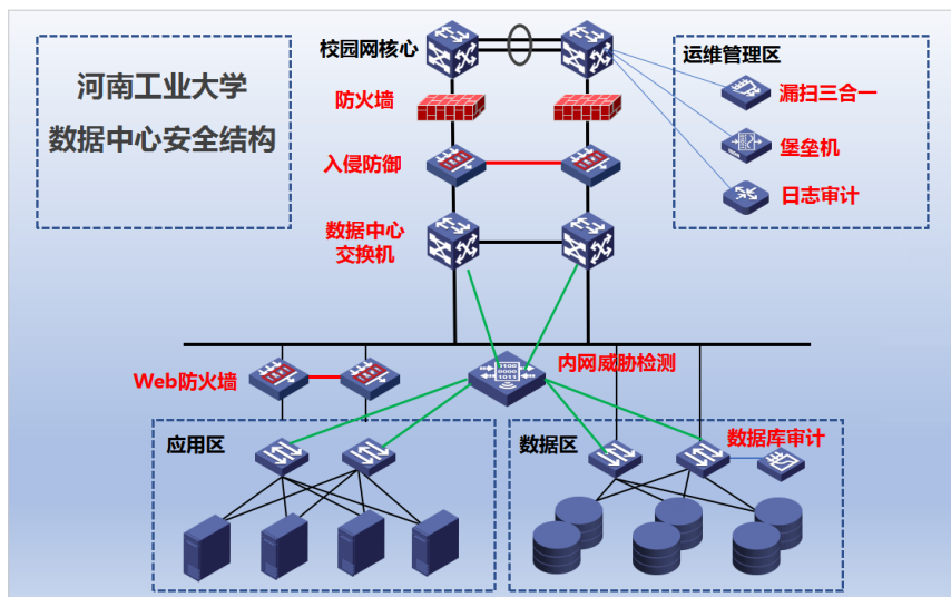
图 1 河南工业大学网络运行与数据安全体系
